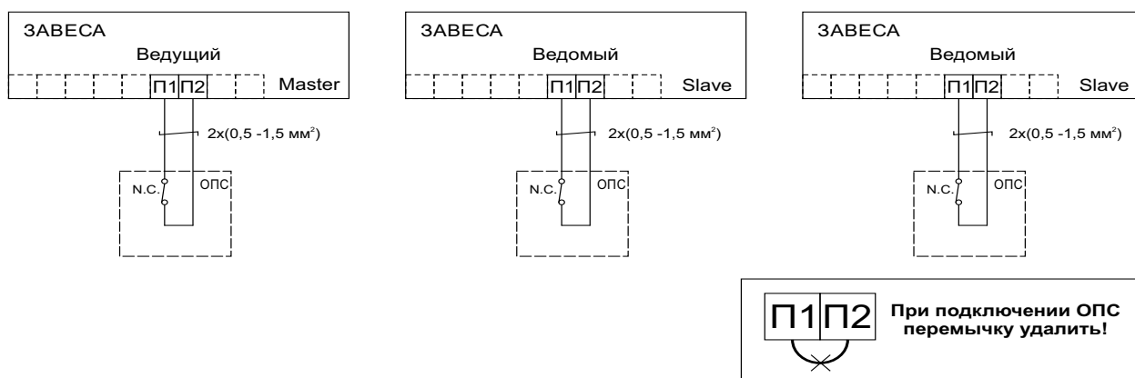
Схема подключения ПКП к группе завес
